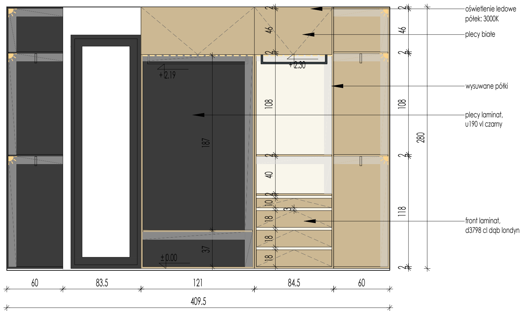
GARDEROBA SYPIALNIA-WIDOK B-B
