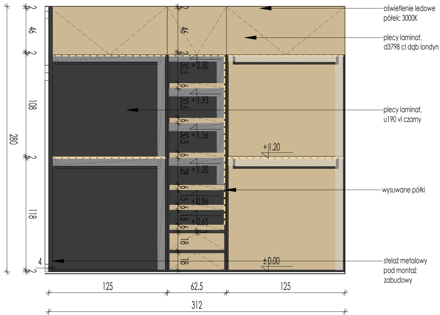
GARDEROBA SYPIALNIA-WIDOK C-C
