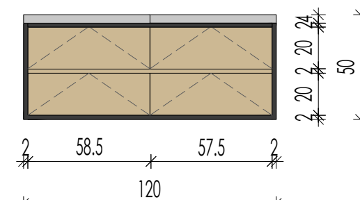
GARDEROBA SYPIALNIA-WIDOK D-D
